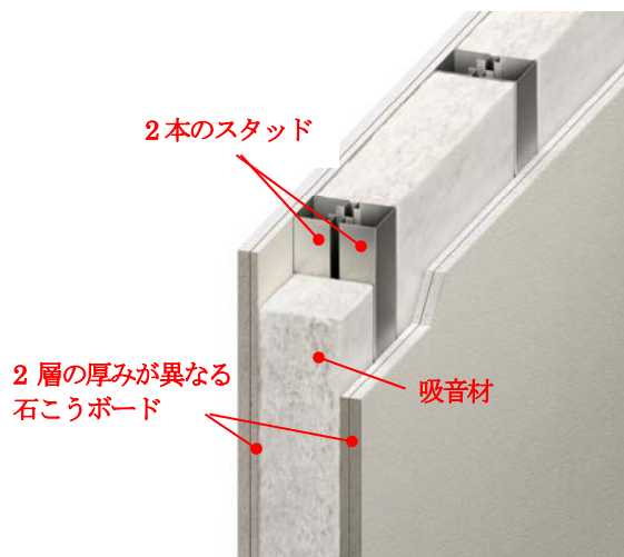
【遮音スタッド界壁 概念図】
