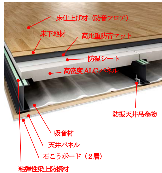
【SR スラブ 55 概念図】
