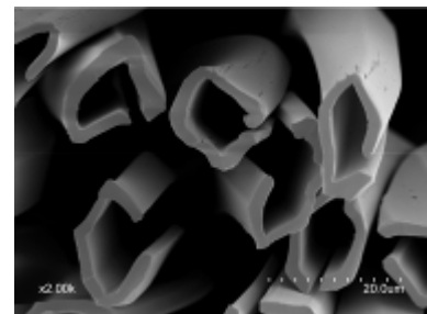
※ミラクルエア断面図
