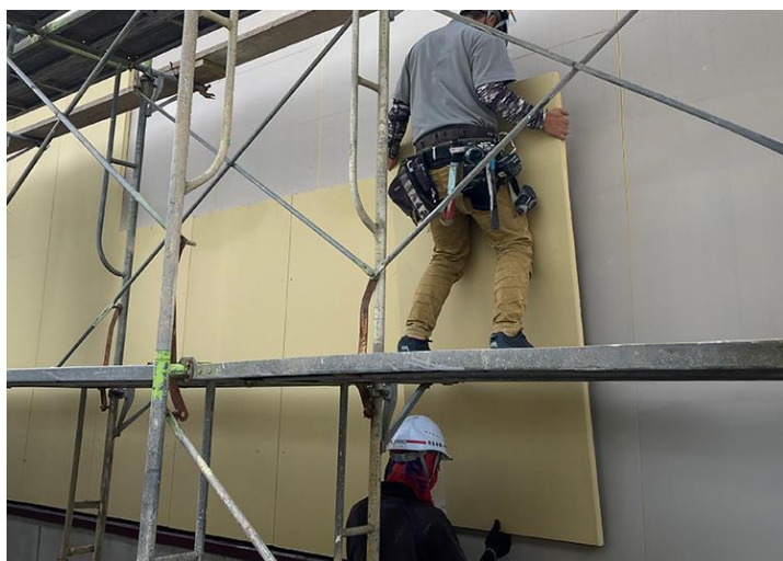
写真:『QD パネル鉄骨外張り断熱システム』施工風景
