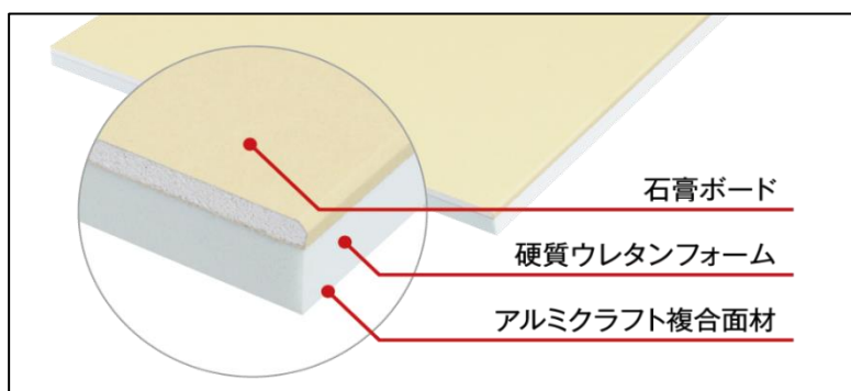
図:『アキレス準不燃 QD パネル』(構造イメージ図)
