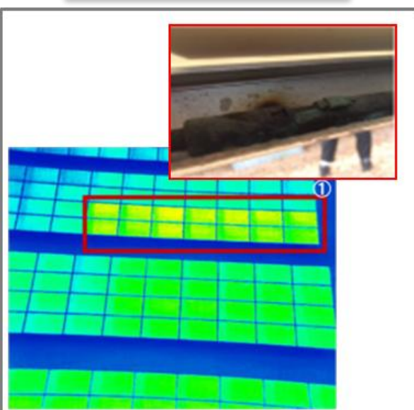
Stringの異常
