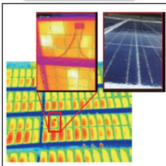
Stringの異常
