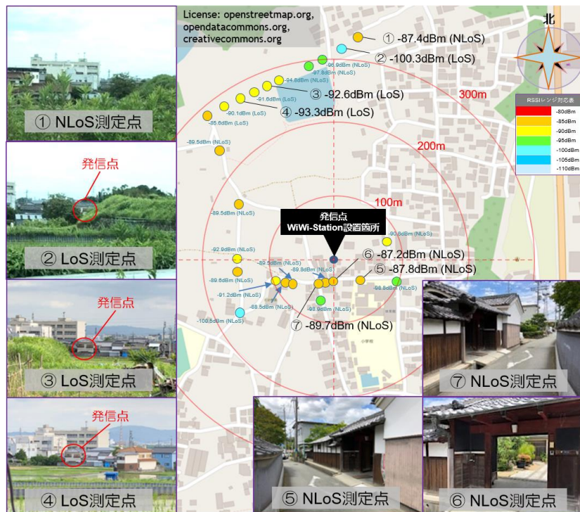
図6 木造家屋にすれ違いIoT無線ルータを設置した場合の通信可能エリア検証結果一例
