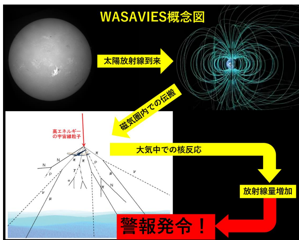
図 3: WASAVIES 概念図
