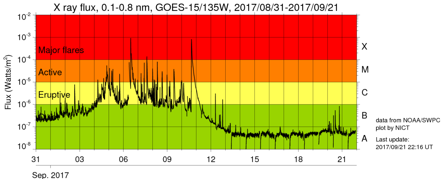
GOES 衛星による太陽 X 線の観測値
