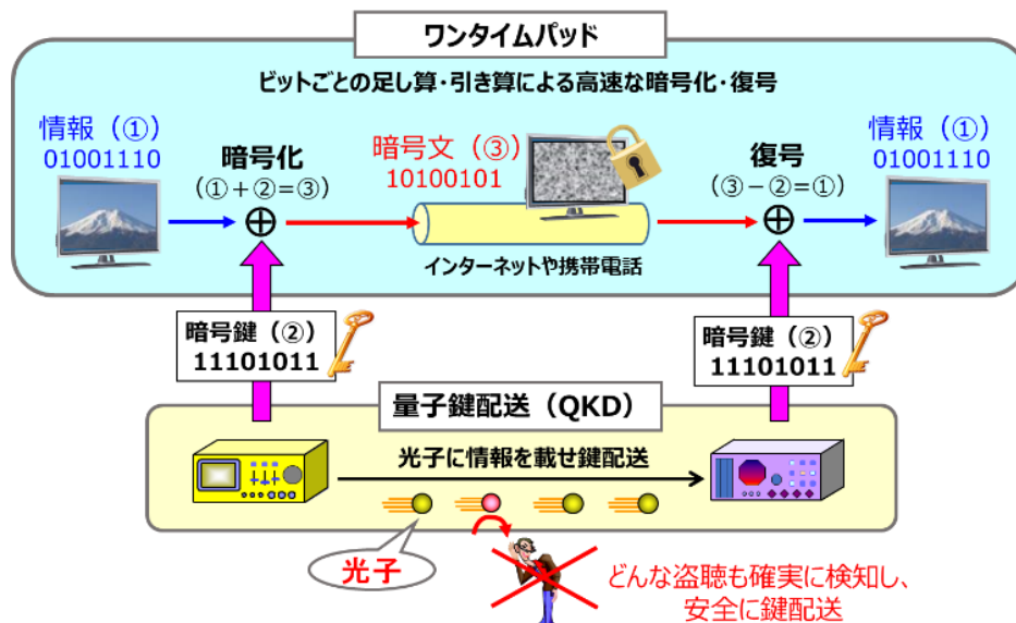
図5 量子暗号模式図
