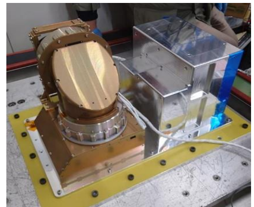
図2 今回開発した SeCRETS のフライトモデル外観
