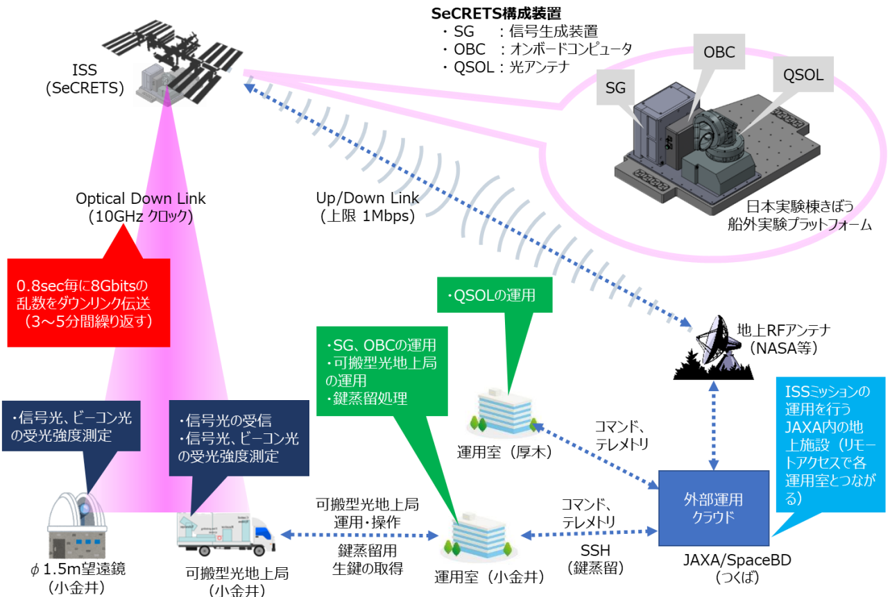
図 1 ISS-可搬型光地上局間の物理レイヤ暗号通信実験の全体構成図
