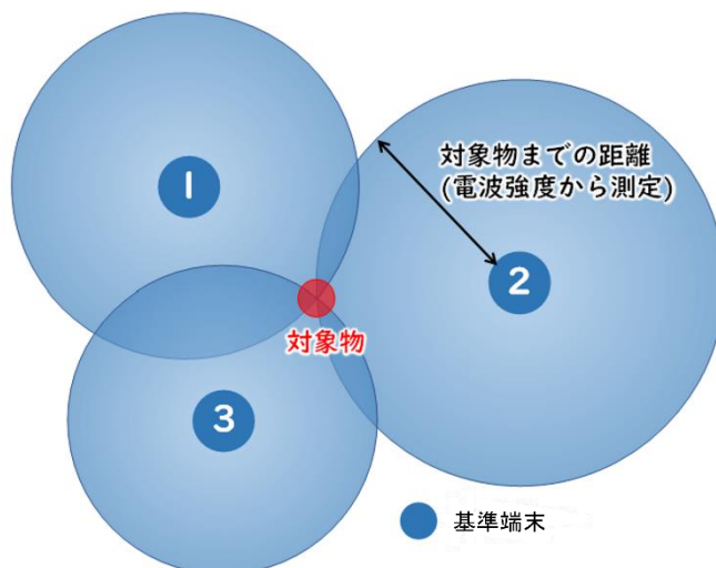
図3 3点測位の原理
