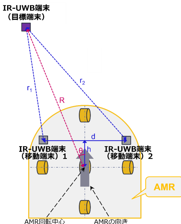
図4 本システムでは目標端末に対する距離計測結果から方向角と距離を計算
