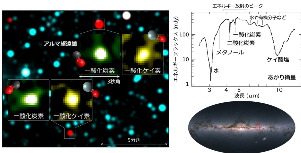
図1. (左) アルマ望遠鏡が捉えた謎の氷天体からの分子輝線放射。背景の画像は、波長 1.2\ \mu\text{m} の光を青で、 4.5\ \mu\text{m} の光を赤で色付けした赤外線カラー合成図 [2MASS および WISE 注5 による赤外線データに基づく]。(右上) あかり衛星により観測された左図上側の天体の赤外線スペクトル。氷や塵による吸収バンドが見られます。(右下) 2つの氷天体の銀河面上での位置 (ESA/Gaia/DPAC の画像を改変)。クレジット：ALMA (ESO/NAOJ/NRAO) , Shimonishi et al. , ESA/Gaia/DPAC
