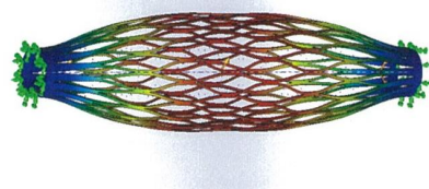
図3. 生体用ステントの拡張時をシミュレーションした画像
