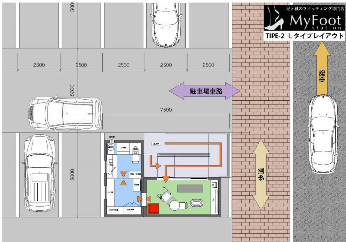
「My Foot Station MINI」の配置図（接客スペース+作業スペース）
