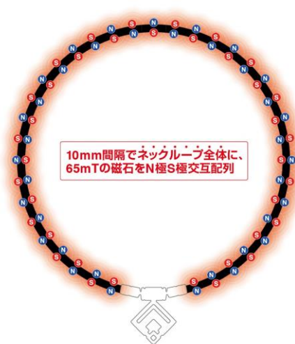
磁石配置図
