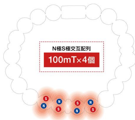
磁石配置図
