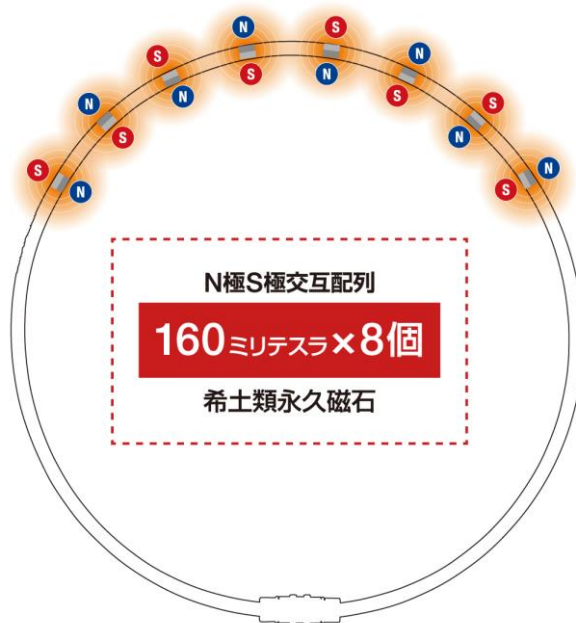
磁石配置図
