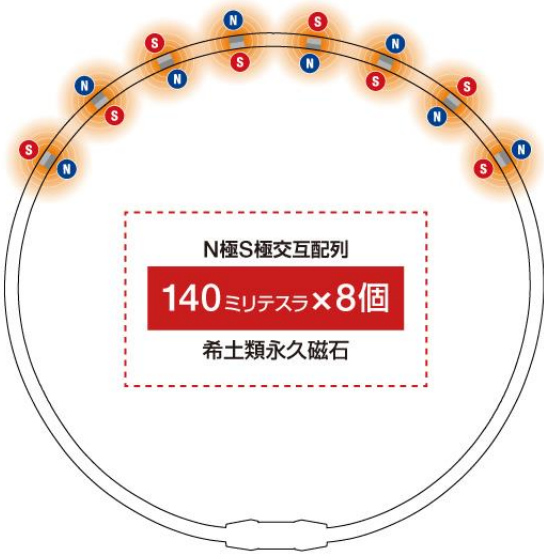
磁石配置図
