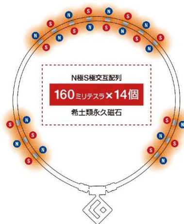
磁石配置図
