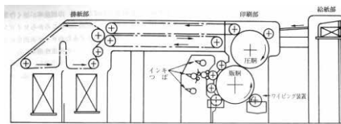
ドイツ製のジオリ4P凹版輪転印刷機（凹版ザンメル印刷）とその構造図
