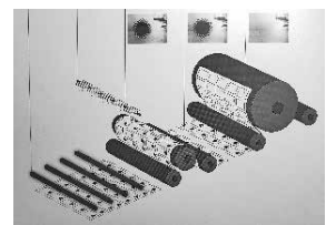
(図版) OVI (光学的变化インキ) の磁性付与の 印刷工程 (SICPA 社のパンフレットより引用)
