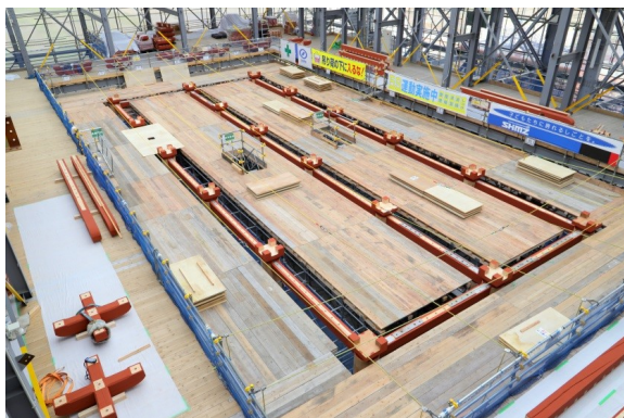
令和元年 7 月 9 日頭貫
