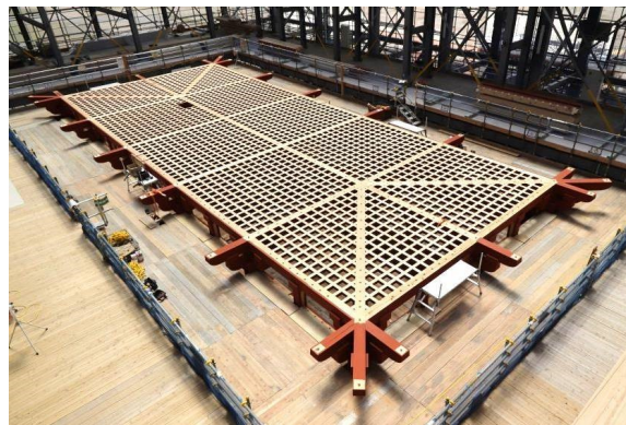
令和元年 8 月 5 日天井格子
