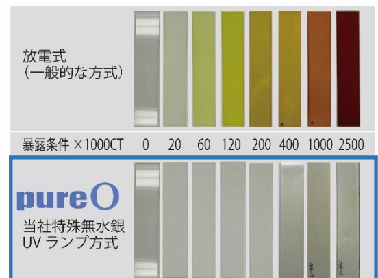
社内暴露試験結果 (ポリウレタンゴム)
