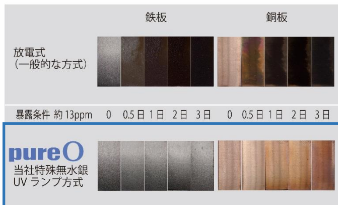
社内暴露試験結果 (鉄板・銅板)
