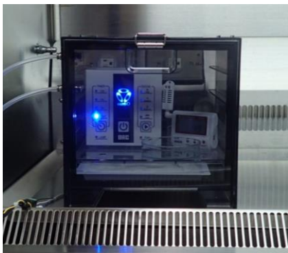
本研究における試験の様子。左：デシケーター内でのオゾン曝露の様子。右：オゾン濃度モニターによるオゾン濃度の制御。
