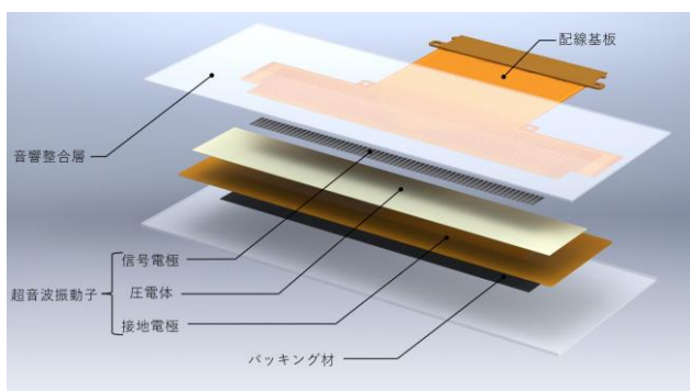
ウェアラブルエコーセンサ 構成図
